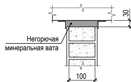
Примыкание перегородки к потолку
