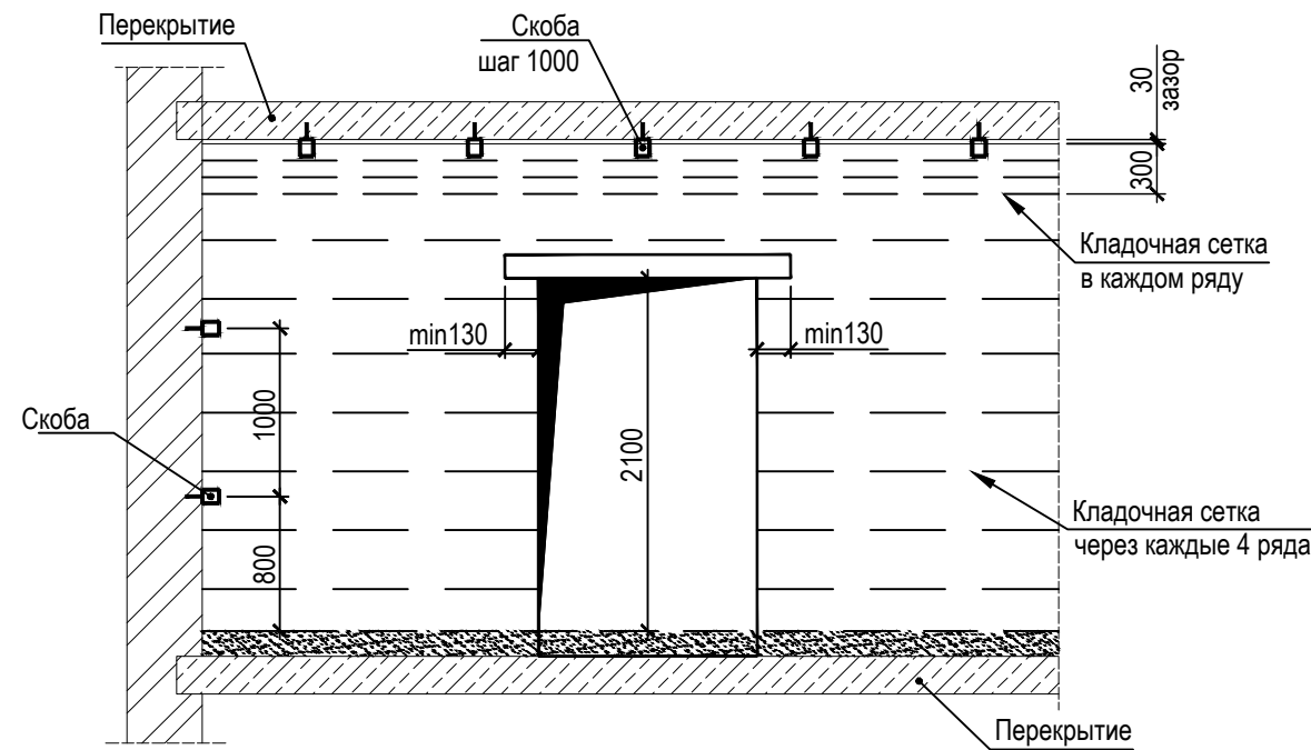
Примыкание перегородки к стене
