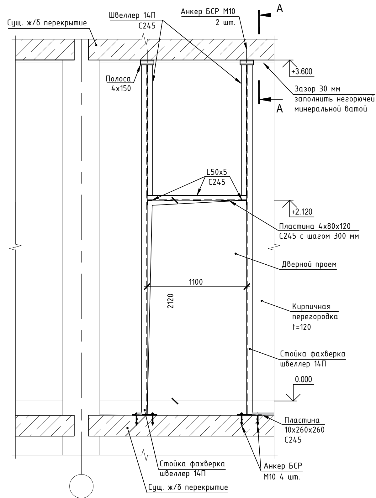
Схема устройства конструкций фахверка перегородки в местах установки противопожарной двери
