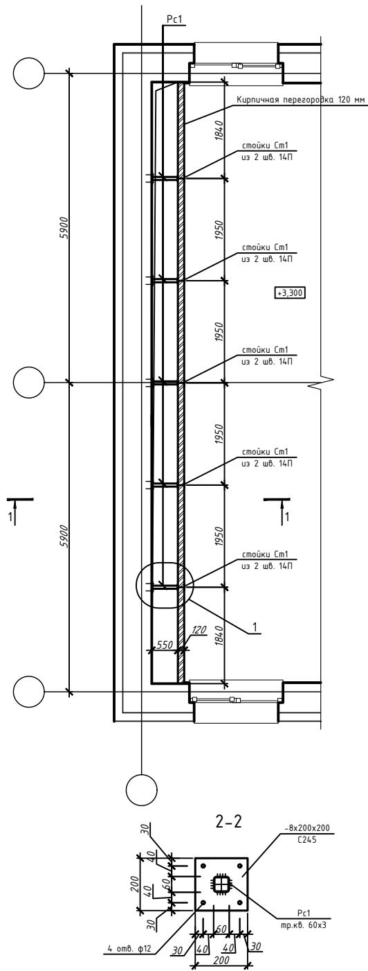
Схема устройства конструкций фахверка кирпичной перегородки
