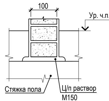
Опираение перегородки
