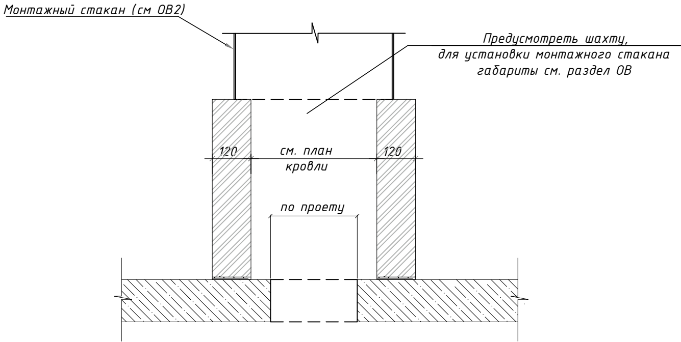
Схема устройства вентиляционной шахты для установки монтажного стакана
