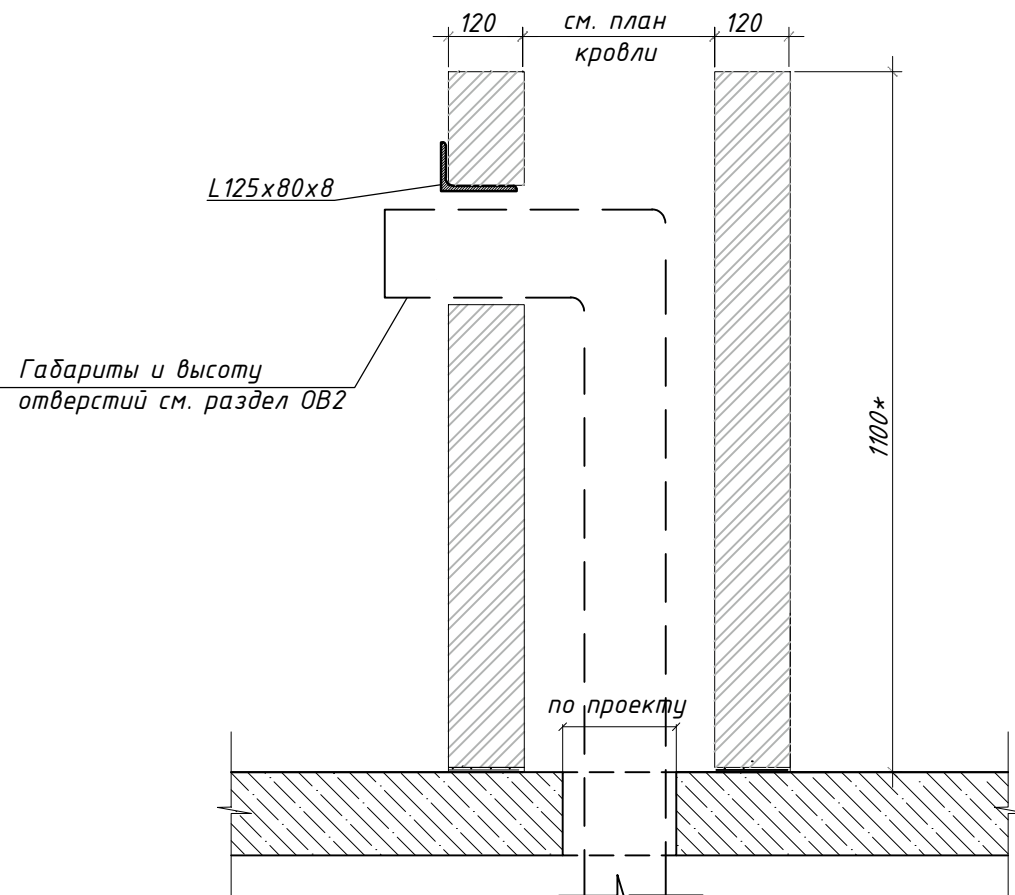
Схема устройства вентиляционных шахт с доковым проходом
