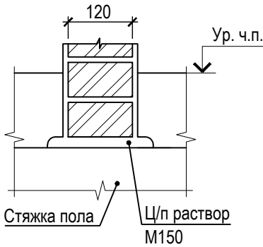
Опираение перегородки
