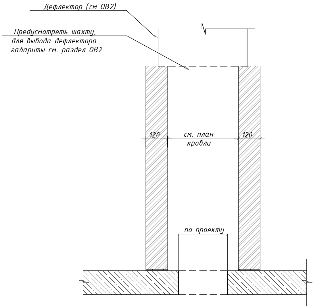
Схема устройства вентиляционной шахты с открытым верхним оголовком
