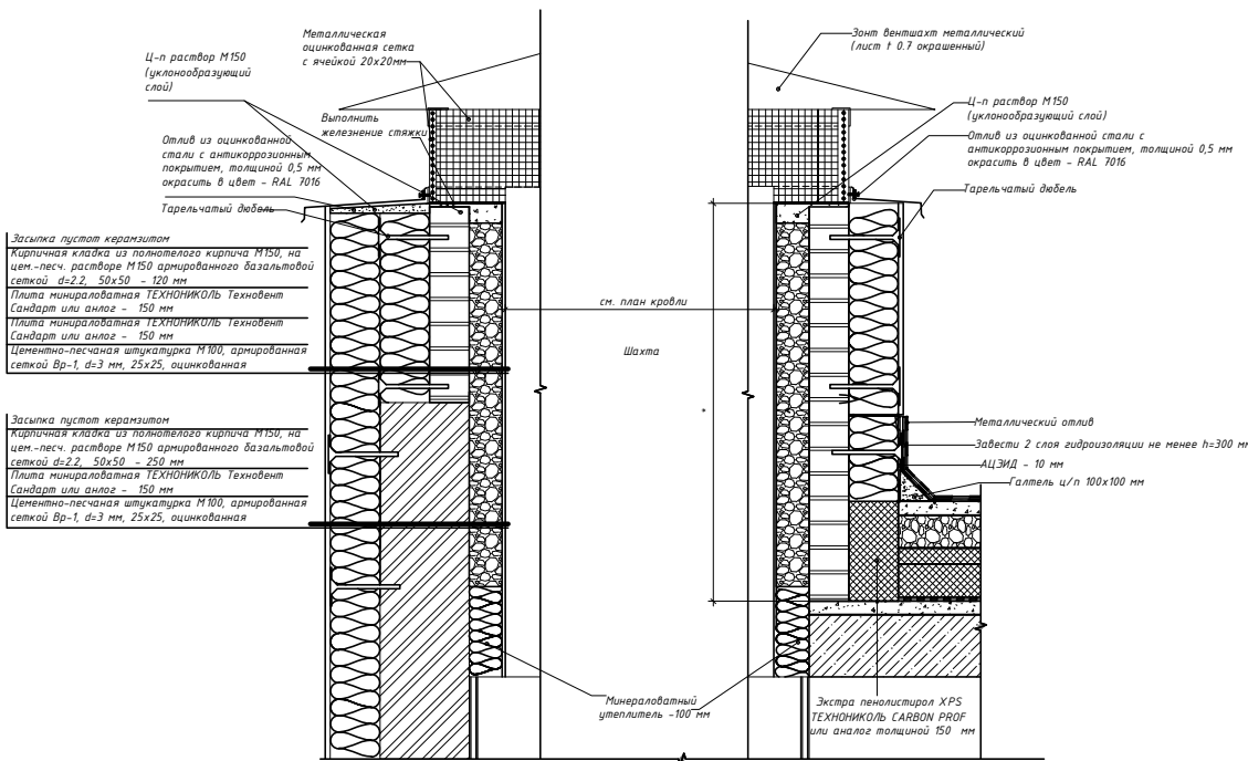
Узел устройства шахт, примыкающих к парапету
