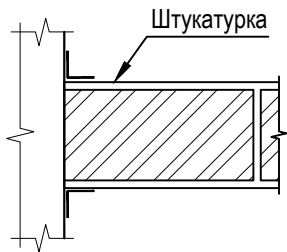
Примыкание перегородки к стене
