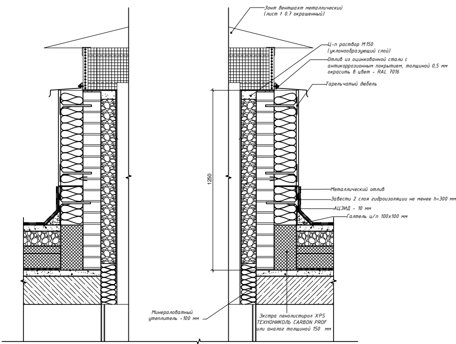
Узел устройства отдельностоящих вентшахт на кровле
